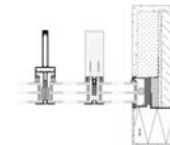
Gläser mit Statiklisene: Außen Alu schwarz eloxiert innen nach Wahl in Holz in der Fensterfarbe oder als schlankes Aluminiumprofil nach RAL
